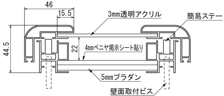
断面A-A'
