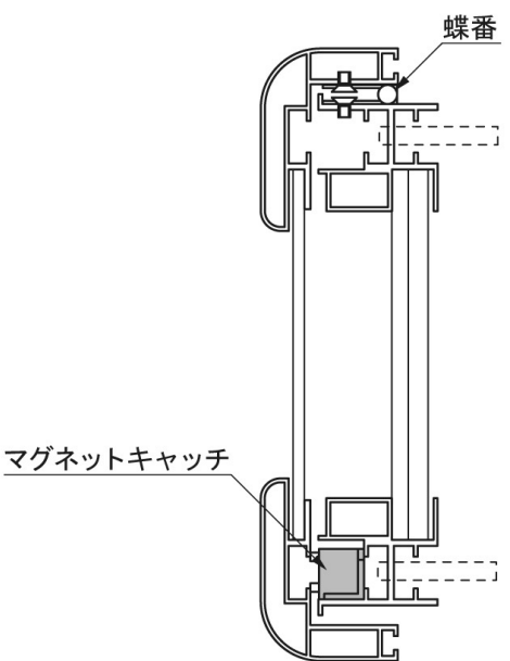
断面B-B'
